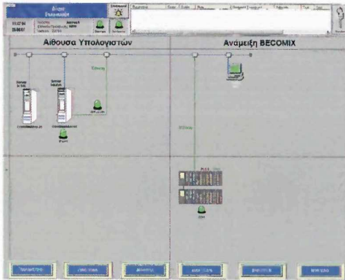
Visione d'insieme generale del sistema. Le connessioni fra i PLC e il Becomix mixing PC vengono raccolte dai server
